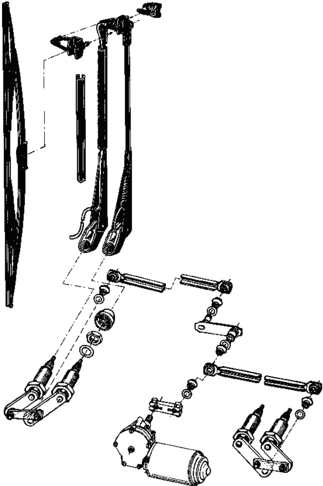
Prinziple sketch
